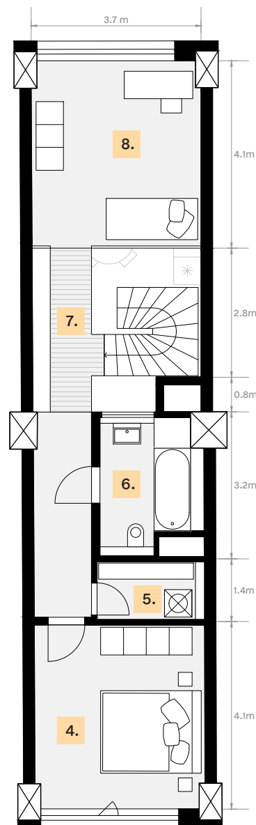
Vrchné podlažie
